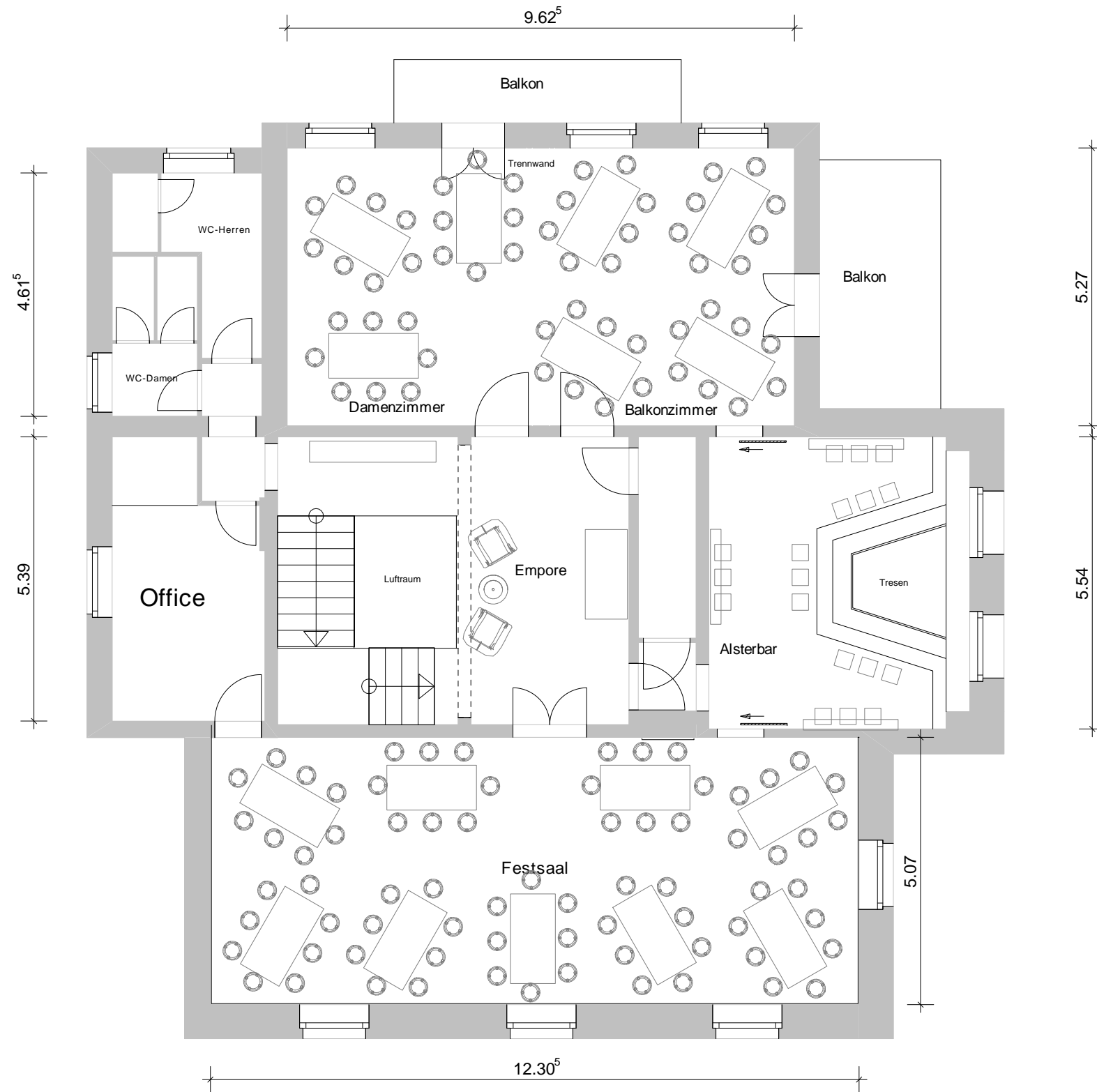
1. Obergeschoss Variante 2
